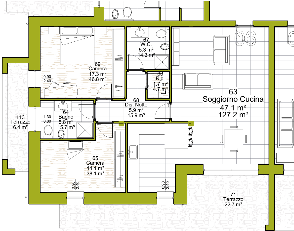
App 06 Scala 1 : 100
